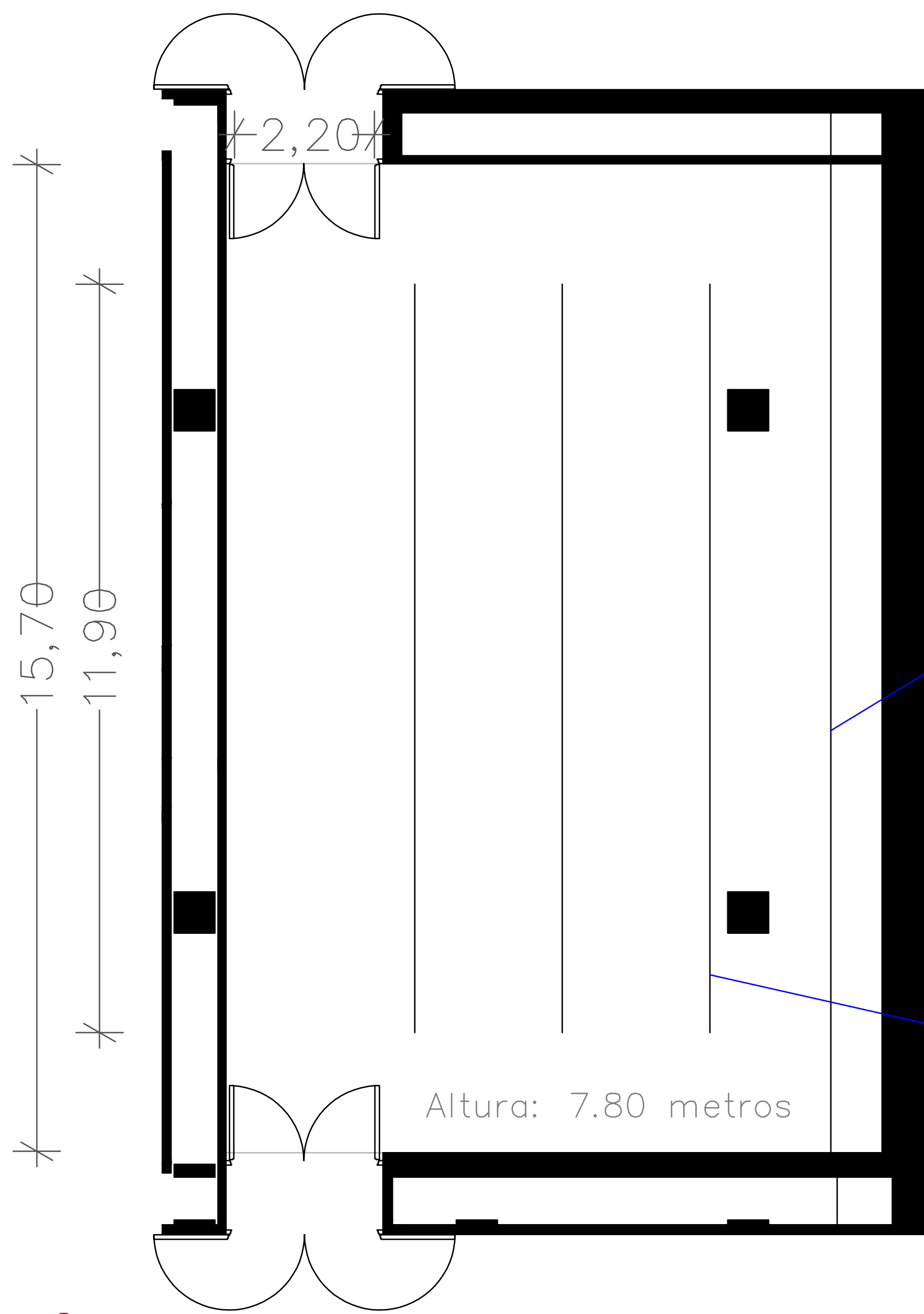
Planta 2
